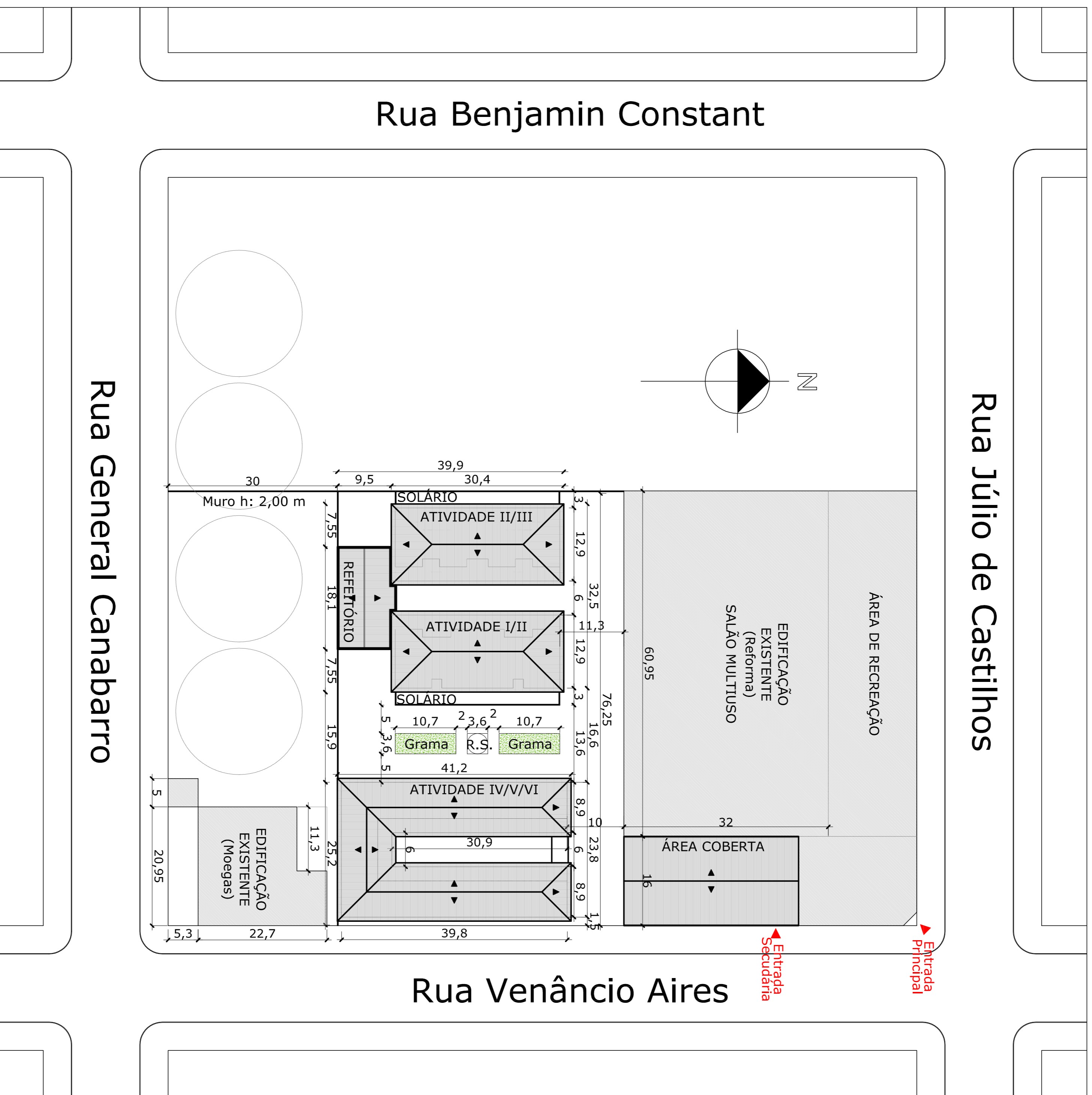
PLANTA DE SITUAÇÃO Escala: 1/500
